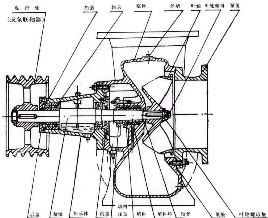
图 1 100~350HW 型泵结构图 (350HW—8 泵有向上和水平两种出水型式)
