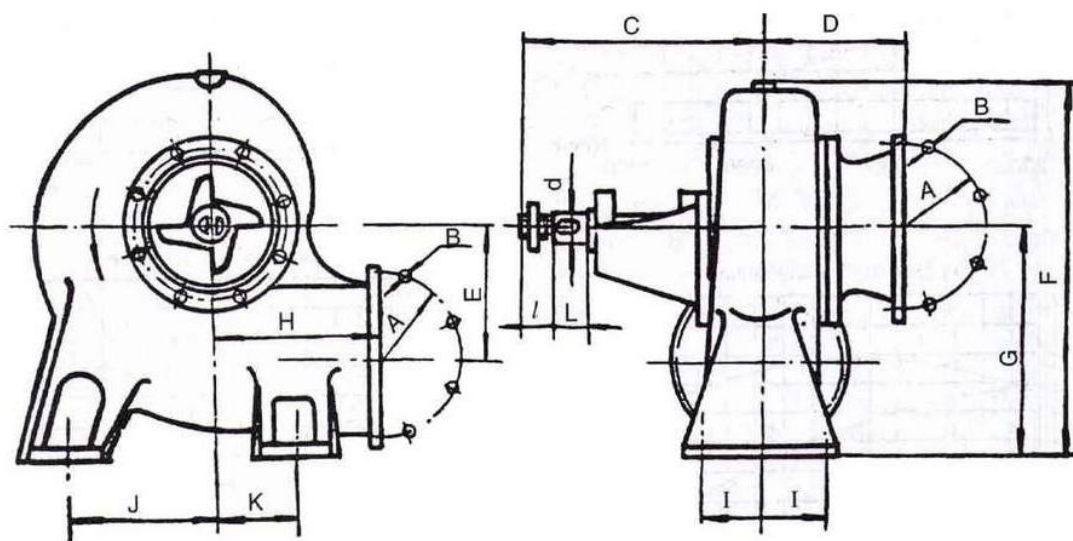
图5 400HW ~ 800HW和350HW-8泵水平出水外形安装图(650HW型泵的出水方向和叶轮转向与图示相反。)
