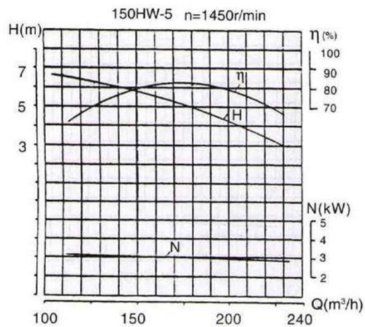
HW 型泵工作性能曲线
