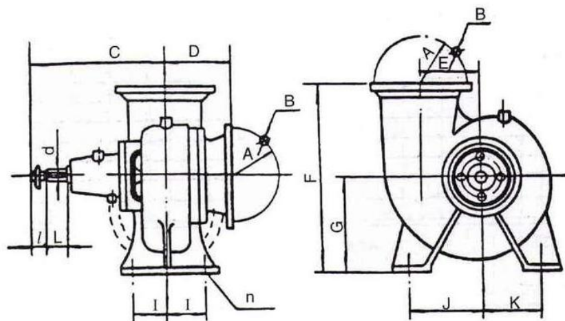
图4 150HW ~ 300HW和350HW-8泵向上出水外形安装图
