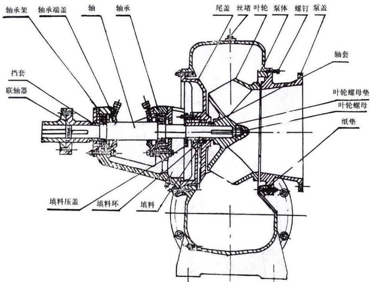
图2 400~800HW 型泵结构图(650HW-5、-7、-10 型泵的出水方向与图示相反 ——向泵进口看, 叶轮为顺时针旋转)
